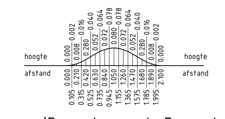
Dwarsdoorsnede Drempeel 20 km/uur Schaal 1:50
