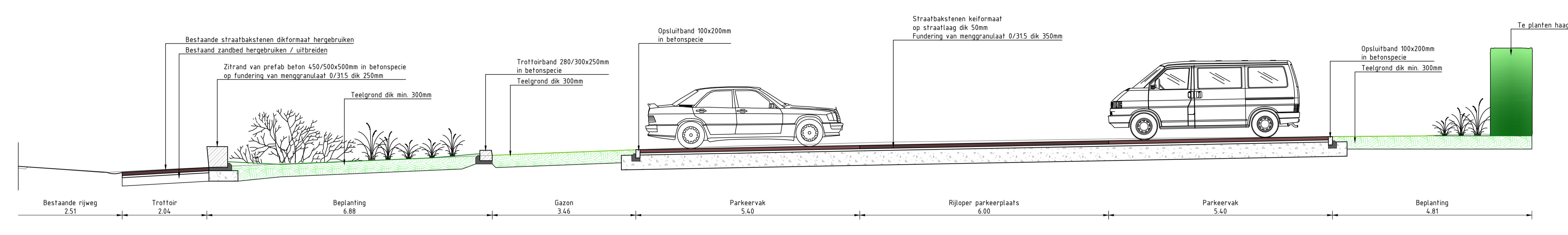
Normaalprofiel A-A Schaal 1:50
